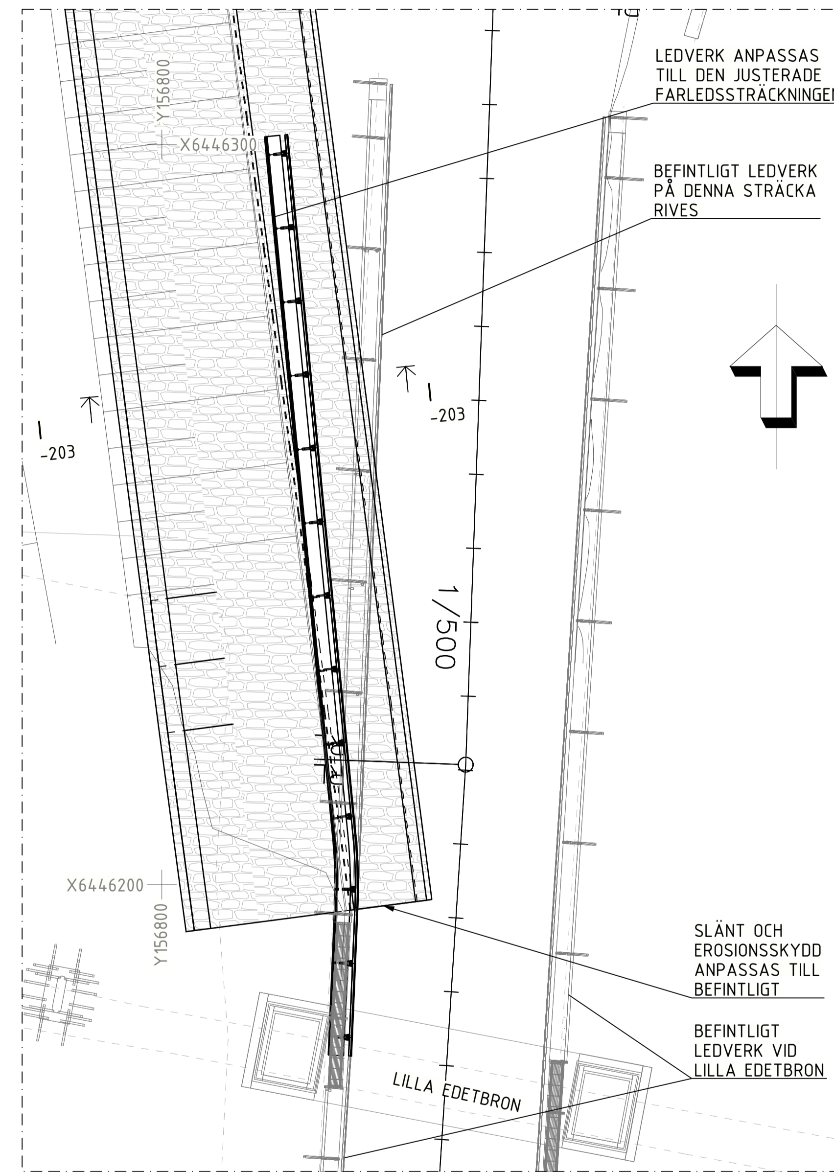
PLAN, UTVINKLAT LEDVERK 1:500
